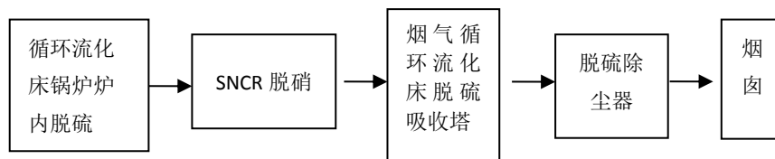
图 D.4 以烟气循环流化床作为炉后脱硫工艺的循环流化床锅炉典型超低排放技术路线
