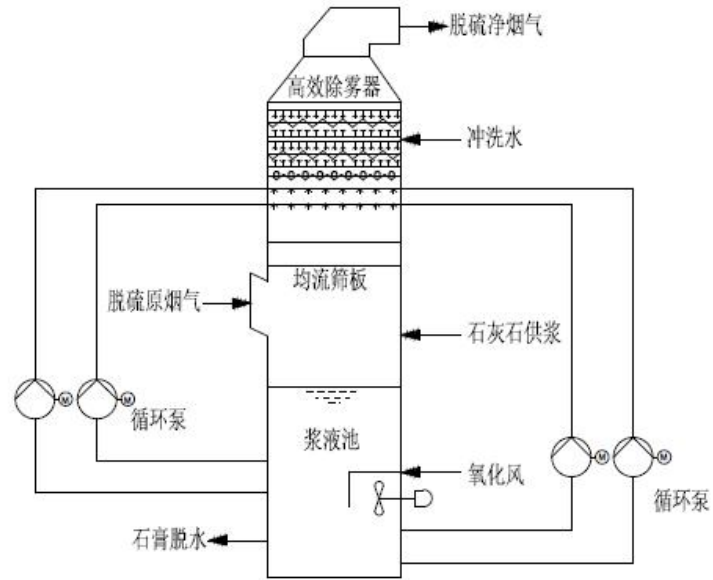
图 H.5 典型石灰石-石膏湿法均流筛板持液脱硫工艺流程
