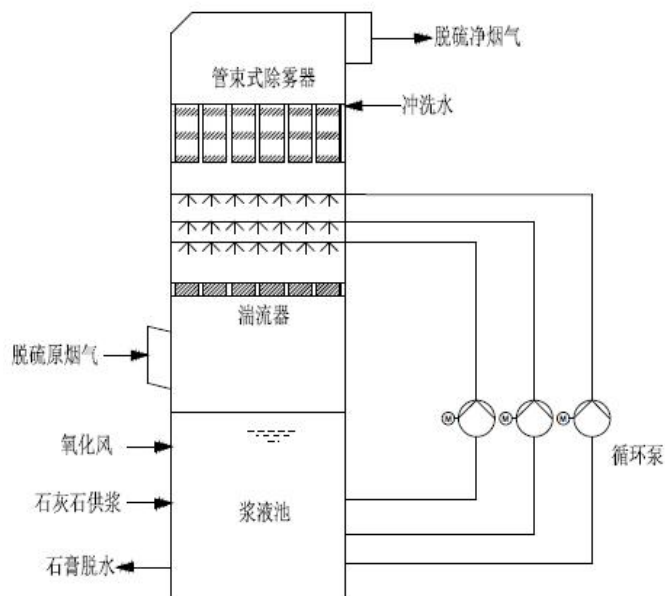
图 J.4 典型石灰石-石膏湿法湍流器持液脱硫工艺流程
