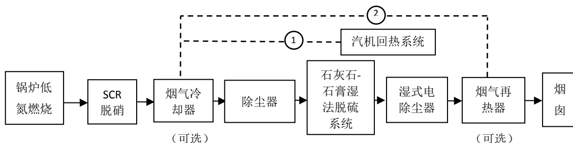
图 D.1 以湿式电除尘器作为二次除尘的典型超低排放技术路线
