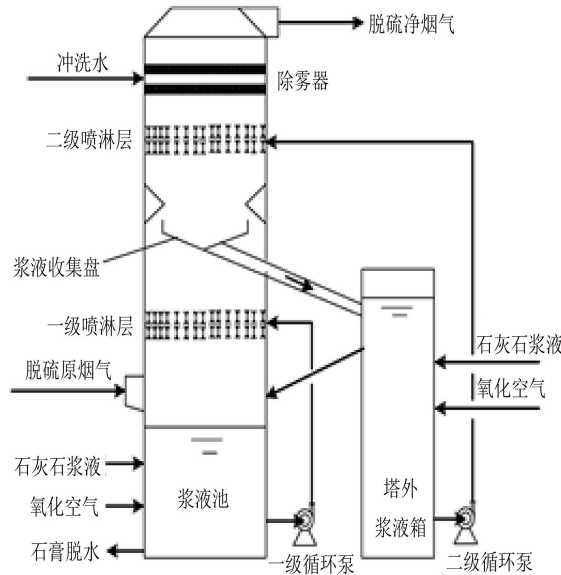
图 H.1 典型石灰石-石膏湿法 pH 值物理强制分区双循环脱硫工艺流程
