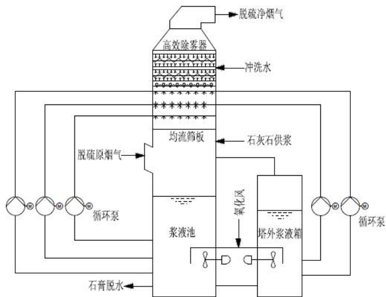
图 J.3 典型 pH 值物理强制分区脱硫工艺流程
