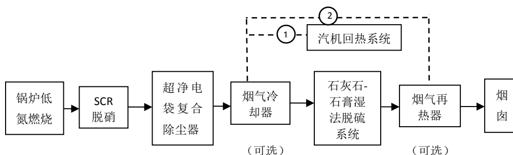
图 D.3 以超净电袋复合除尘器作为一次除尘且不依赖二次除尘的典型超低排放技术路线
