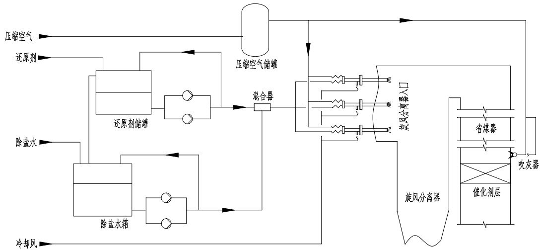
图3 典型循环流化床锅炉SNCR/SCR联合脱硝工艺流程
