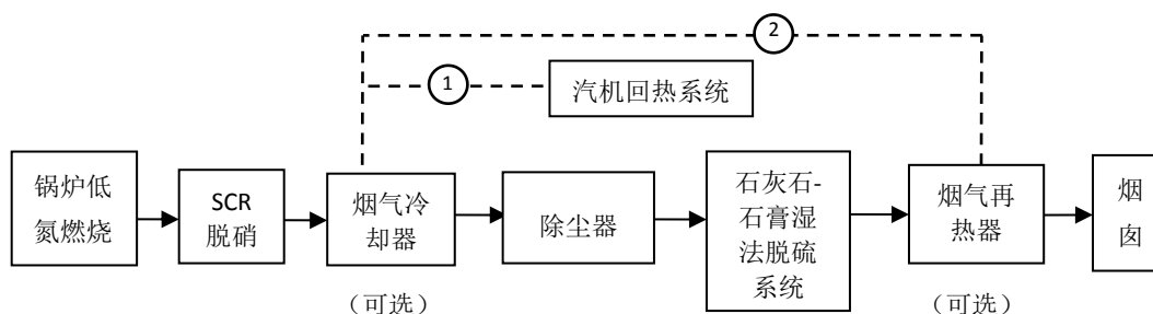
图 D.2 以湿法脱硫高效协同除尘作为二次除尘的典型超低排放技术路线
