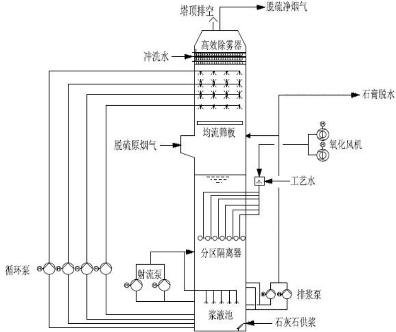
图 J.2 典型石灰石-石膏湿法脱硫 pH 值自然分区脱硫工艺流程
